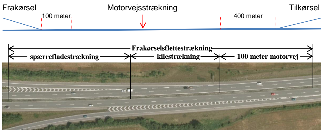
Figur 1. Definition af motorvejs- og frakørselsflettestrækning til uheldsmodellering.
