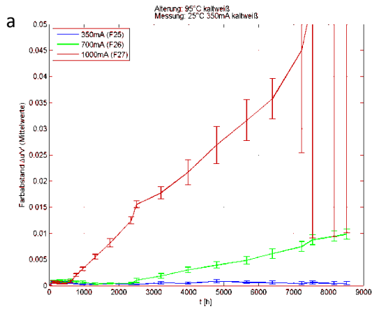
Abbildung 2.17: LED2 kaltweiß (a) und warmweiß (b) - Vergleich Farbabweichung über die Zeit
