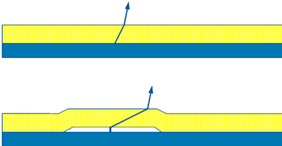
Abbildung 2.48: Strahlengang des blauen Lichts in der LED Oben: normale LED Unten: delaminerte Leuchtstoffschicht
