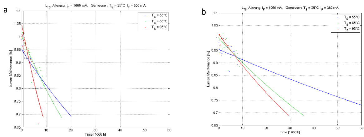
Abbildung 2.22: LED1 kaltweiss (a) und warmweiss (b) - Alterung mit 1000 mA
