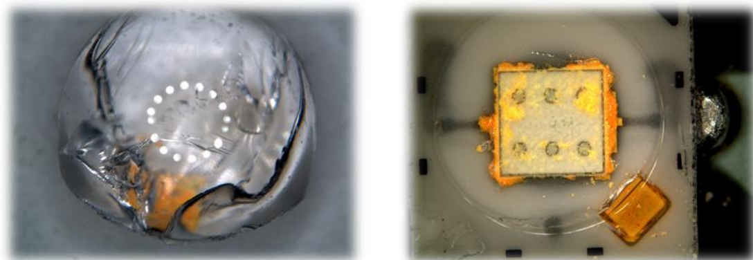
Abbildung 5.9: Gealterte LED an der Hochschule Hannover
