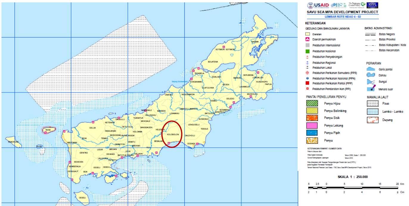
Gambar 1. Lokasi pengamatan vegetasi di Desa Kolobolon, Kecamatan Lobalain, Rote Ndao
