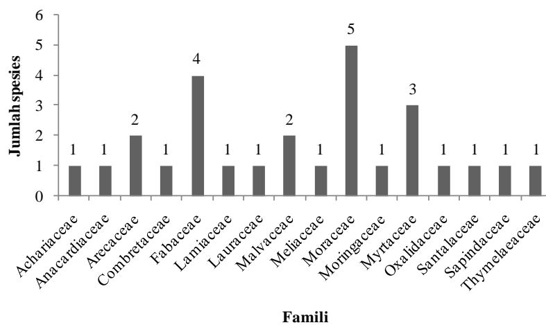
Gambar 2. Jumlah spesies vegetasi pohon berdasarkan famili di Desa Kolobolon
