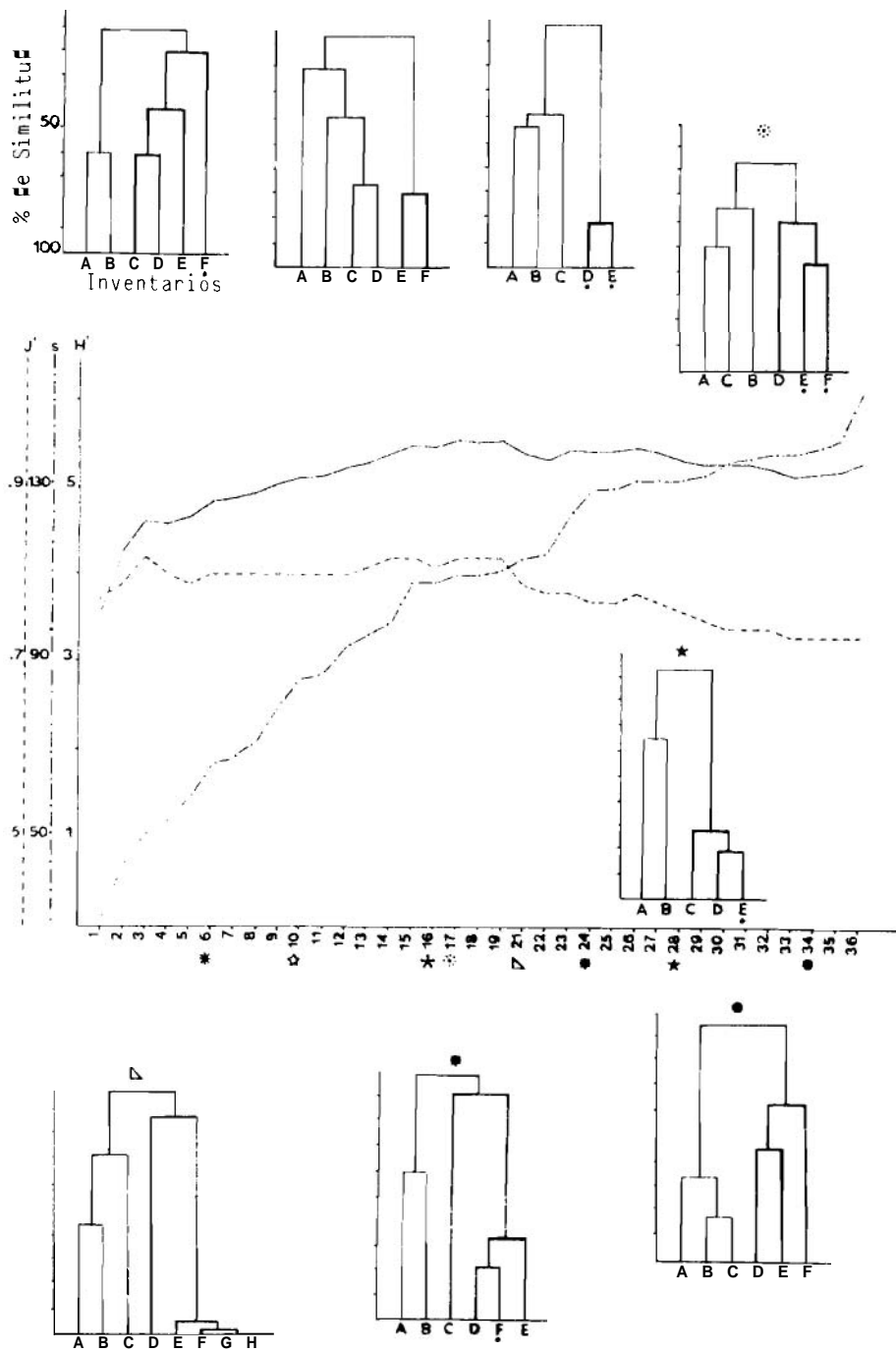
FIGURA 4. Evolución de la diversidad de tipo gamma acumulada para los 36 transectos (inventarios sometidos a una influencia más directa del agua) a lo largo del río. Los inventarios señalados con (.) se sitúan dentro del agua.
