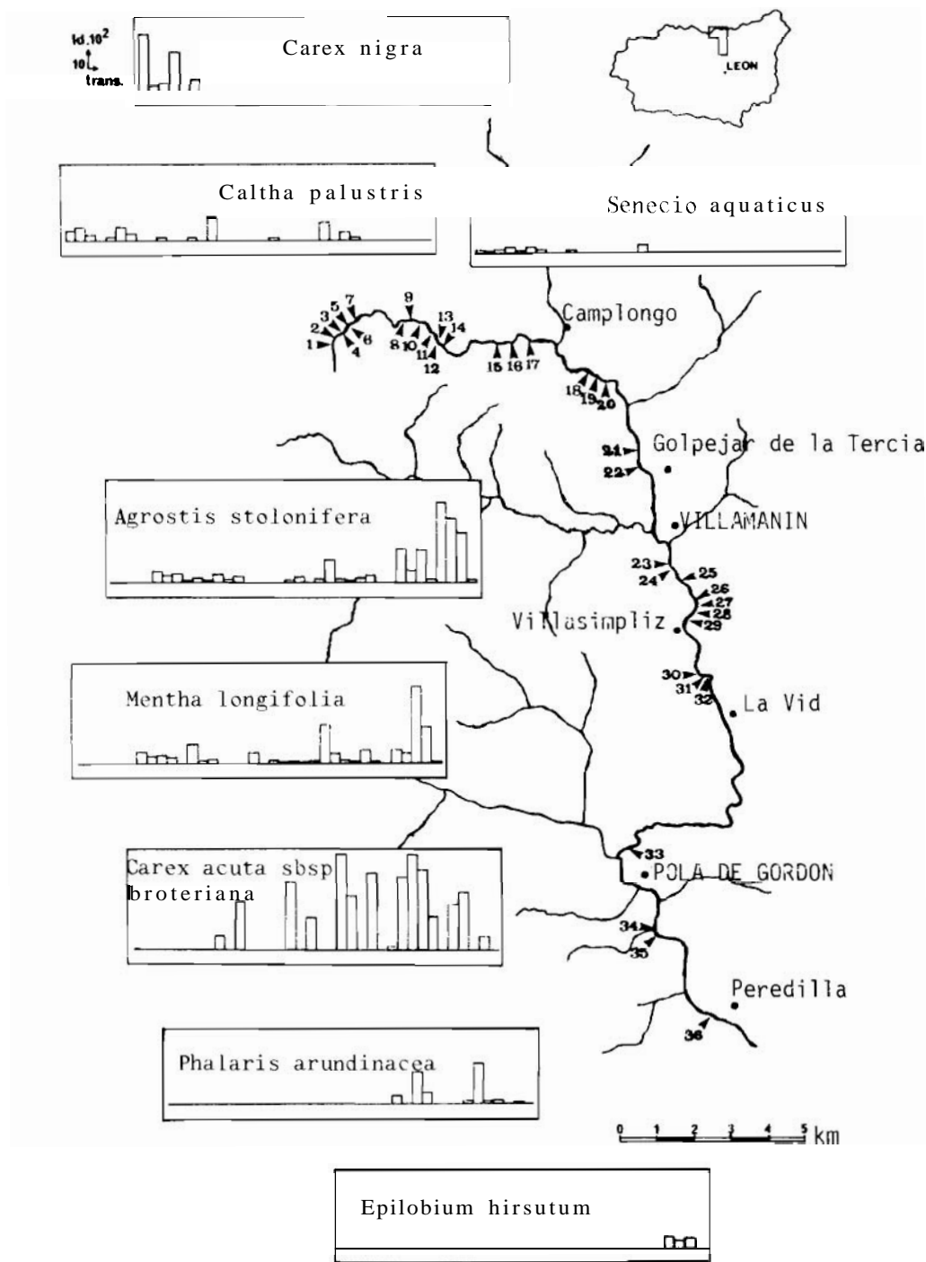
FIGURA 1. Situación de los transectos realizados y distribución de las especies más características a lo largo del río en su tramo de montaña.
