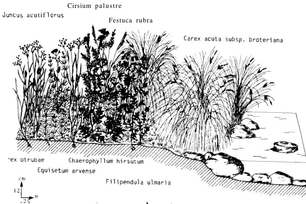
FIGURA 3. Perfil de zonación de la vegetación macrofítica ribereña (Villasimpliz, transecto 28).
