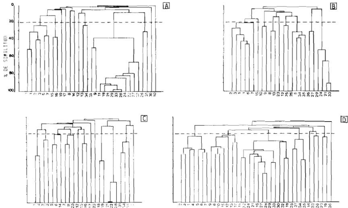
FIGURA 2. Dendrogramas de afinidad entre las muestras situadas a distintos niveles de proximidad al agua (A, a 0 m; B, a 0,5 m; C, a 1 m) y entre la totalidad de los transectos considerando globalmente todos los inventarios de cada uno de ellos (D).
