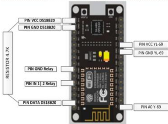
Gambar 2. Konfigurasi Node
