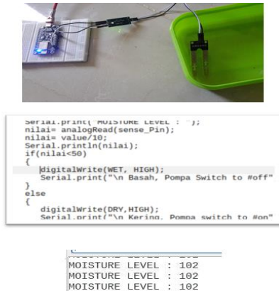
Gambar 6. Pengujian Sensor YL-69
