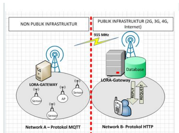
Gambar 1 Konfigurasi Network
