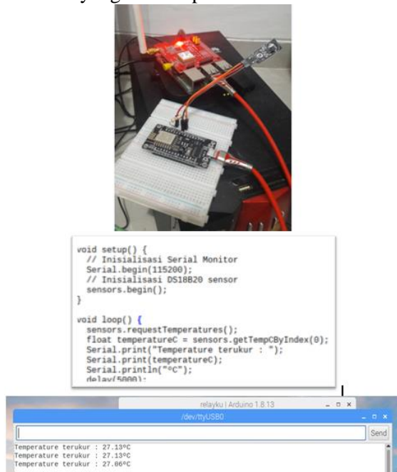
Gambar 7. Pengujian Sensor DS18B20
