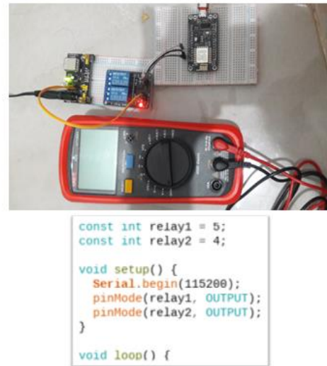
Gambar 8. Pengujian Operasional Relay 5V dengan Eksternal input 5Vdc
