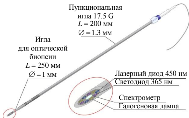
Рис. 8. Опволоконный зонд для оптической мультипараметрической диагностики при проведении чрескожной биопсии
