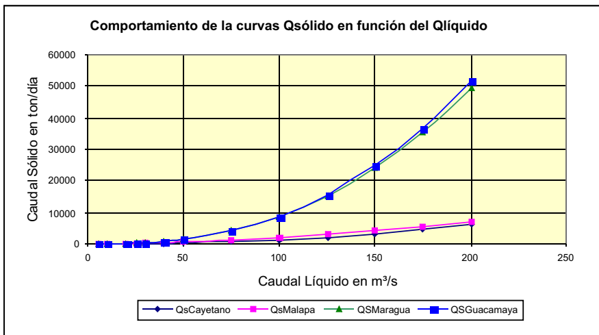
FIGURA 5: Comparación de relaciones QS = f(QL)
