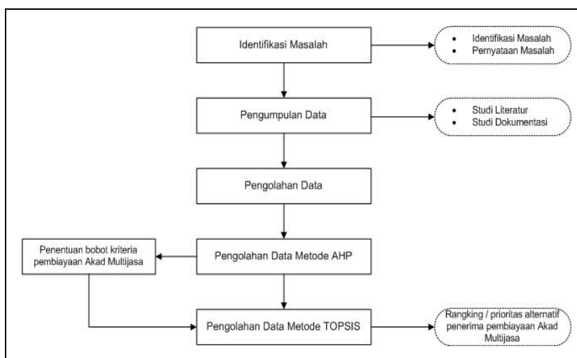
Gambar 1. Tahapan Penelitian
