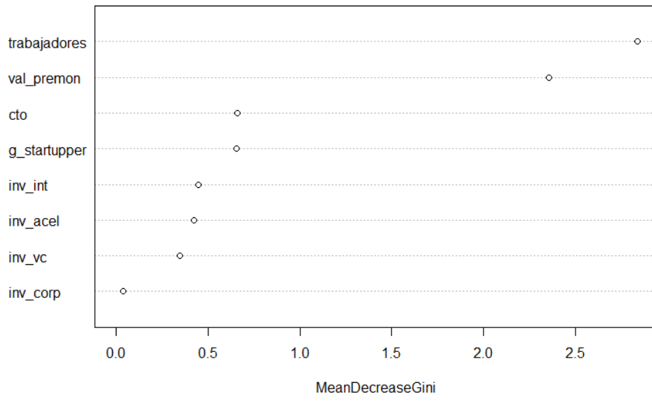
modelo_rf
