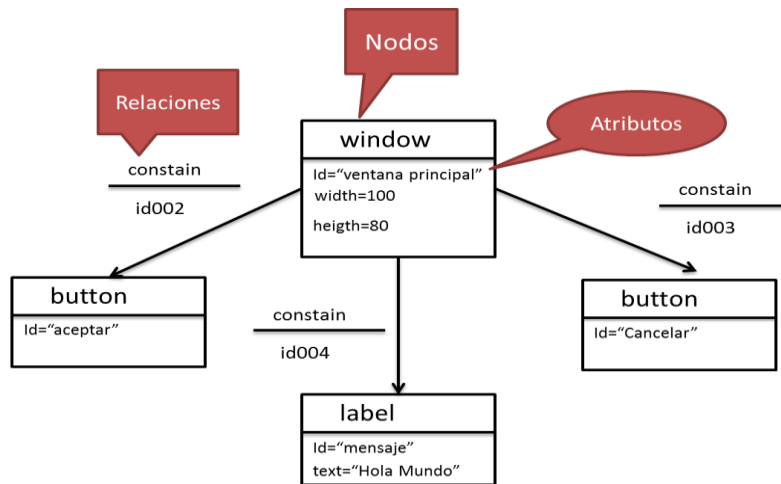
Ilustración 3-6 Representación de una Interfaz de usuario mediante un Grafo
