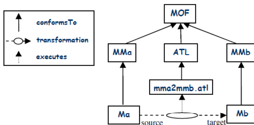
Ilustración 3-4 Enfoque de transformación de ATL
