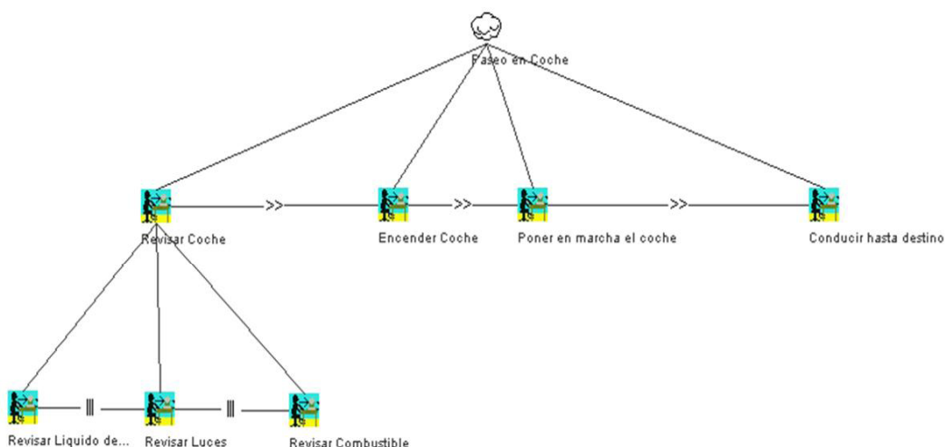
Ilustración 2-6 Descripción jerárquica de un modelo de tareas utilizando la notación CTT
