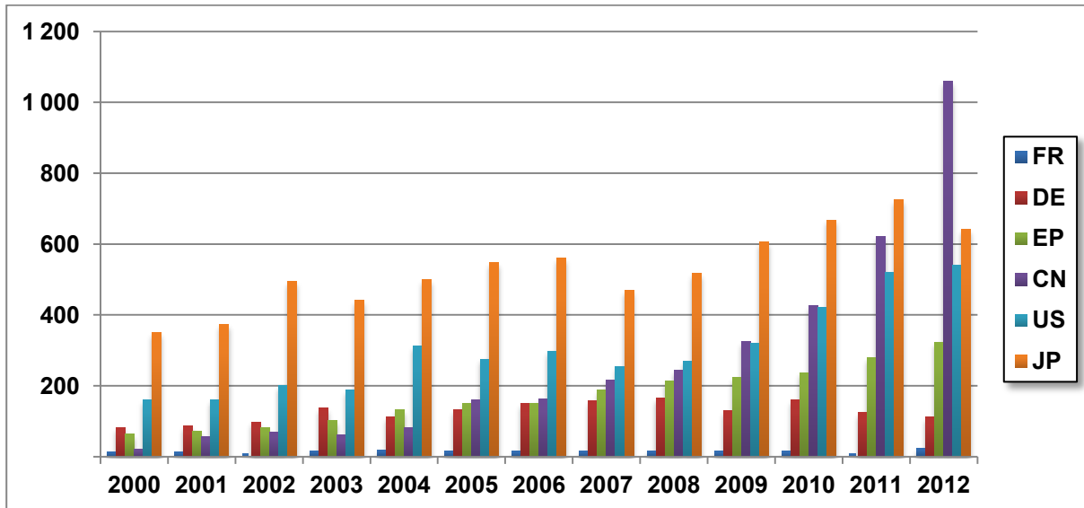
Abb. 4-65 Anzahl Patente im Bereich „Permanentmagnete“ für Synchron-, Reluktanz- und Transversalfflussmaschine nach Weltregionen 2000–2012
