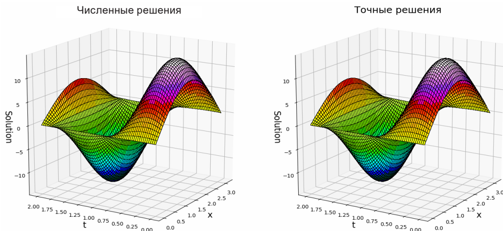
Рис. 3. Численные и точные решения при T = 2 , l = \pi , h = 0,0625 и \tau = 0,03125
