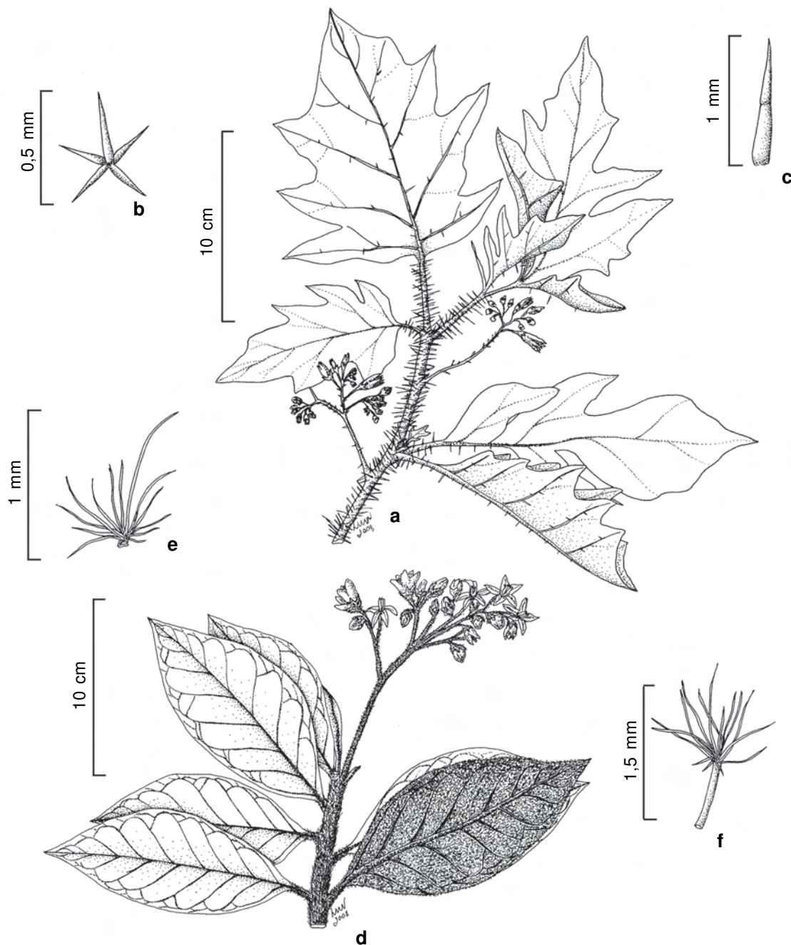
Figura 8 – a-c. Solanum vaillantii – a. ramo com inflorescências; b. tricoma estrelado sésseil; c. tricoma simples; d-f. S. velleum – d. ramo com inflorescência; e. tricoma estrelado ramificado com célula central longa e curva; f. tricoma equinóide (a-c Salimena 2367 ; d-f Abreu 27 ).
