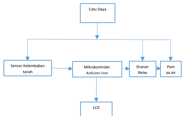
Gambar. 1 Flowchart Keseluruhan Alat
