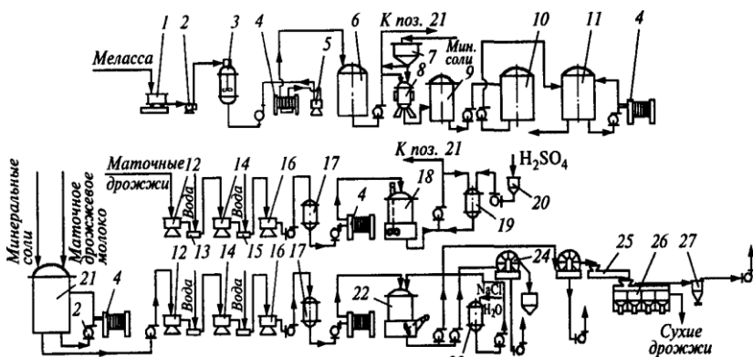
Рис. 10.2. Машинно-апаратурна схема лінії виробництва хлібопекарських дріжджів: збірник меласи 1, насос 2, розсиропник 3, пластинчастий теплообмінник 4, тарифікатор 5, приточний збірник 6, бачок для розчинення мінеральних солей 7, дріжджоростильні апарати (8 — попередній дріжджоростильний апарат; 9, 10, 11 — дріжджоростильні апарати відповідно I, II і III стадії маточних дріжджів), сепаратори 12, 14, 16, промивні бачки 13 і 15, збірник сірчаної кислоти 19, мірник 20, товарний апарат для розмноження дріжджів 21, пластинчастий теплообмінник 22, збірник 23 розчину солі, вакуум-фільтр 24, шнек 25, сушилка для дріжджів 26, циклон 27.
