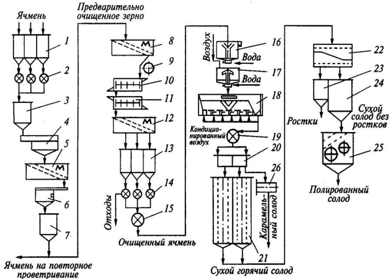
Рис. 7.1. Машинно-апаратна схема виробництва солоду:
