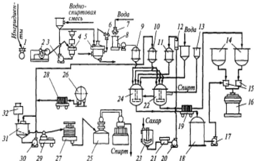
Рис. 8.2. Машинно-апаратурна схема виробництва лікєров та наливков:
