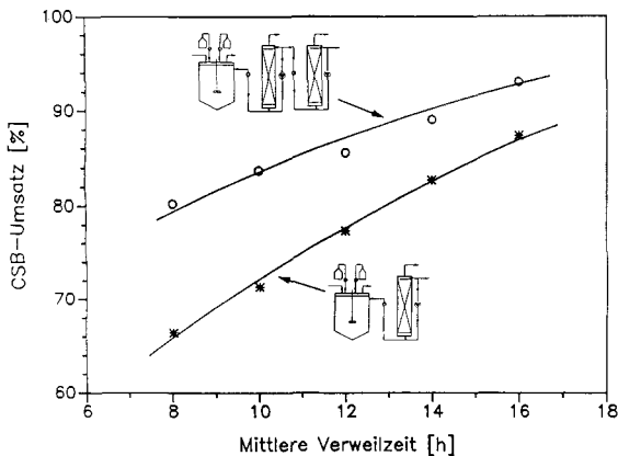
Abb. 2. nderung des CSB-Umsatzes in Abhangigkeit von der Verweilzeit bei der anaeroben Behandlung von Brennereischlempen; Zweistufen-Proze mit und ohne Kaskadenschaltung.
