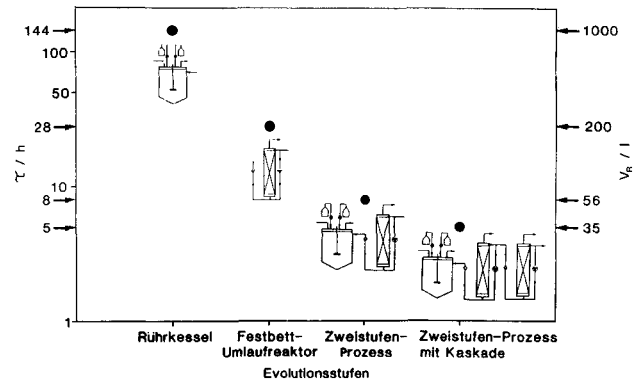
Abb. 3. Entwicklung der minimalen Verweilzeit und des relativen Methanisierungsvolumens fur 85% CSB-Reduktion bei der anaeroben Behandlung von komplex zusammengesetzten Ablufen der Nahrungsmittelindustrie.
