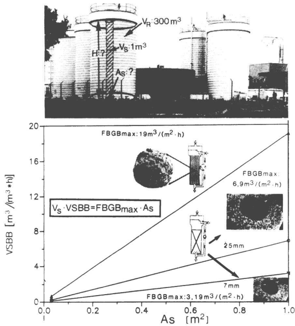
Abb. 1. Vorgehensweise zur Dimensionierung tragerhaltiger Anaerobreaktoren (Festbett-Umlauf- und Wirbelschichtreaktor) auf der Grundlage der maximalen flachenbezogenen Gasbelastung.
