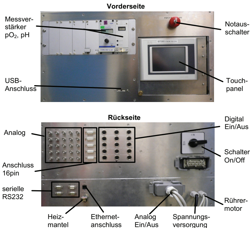
Abbildung 20.1: Vorder- und Rückansicht der entwickelten Steuer- und Regeleinheit für das Reaktorsystem zur Durchführung von 13 C-Markierungsexperimenten
