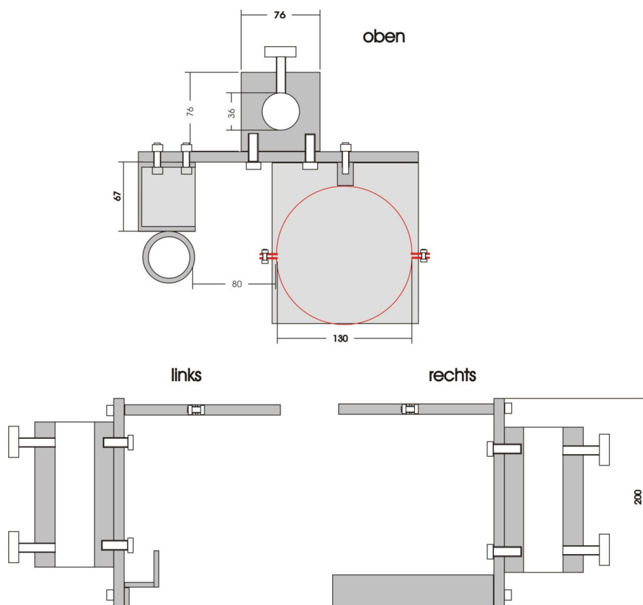
Abbildung 18.7: Maßzeichnung der Halterung für Reaktor und Markierungsaufgabeeinheit
