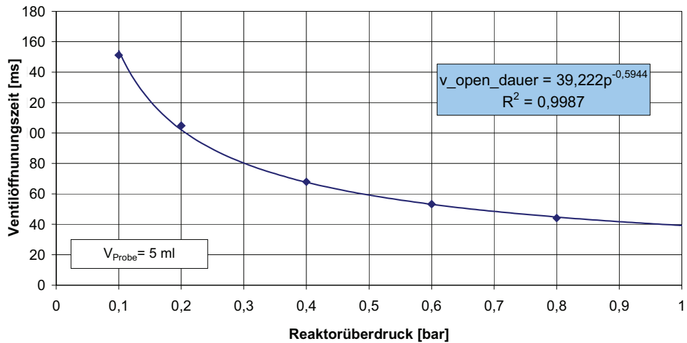
Abbildung 18.9: Abhängigkeit der Ventilöffnungszeit vom Druck für 5 ml Probevolumen
