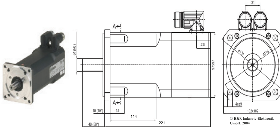
Abbildung 18.6: Foto und Maßzeichnung des B&R-Motors 8MSA4.E0-00
