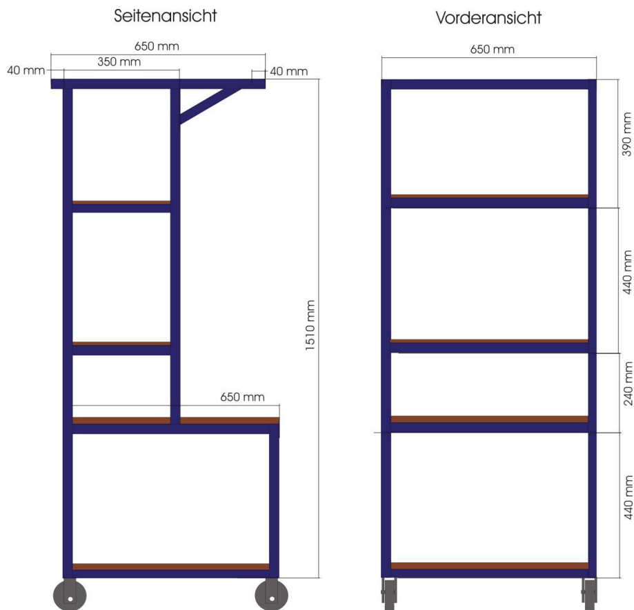
Abbildung 19.1: Maßzeichnung des Stahlrohrgestells für das Reaktorsystem
