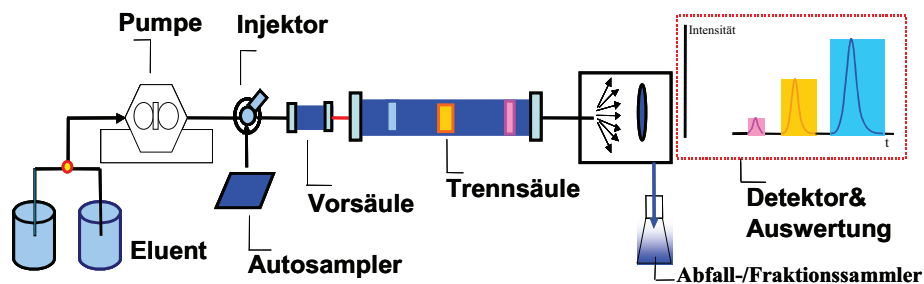
Abbildung 6.1: Funktioneller Aufbau einer HPLC-Anlage
