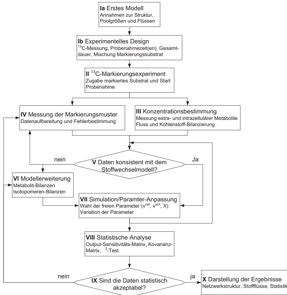
Abbildung 7.5: Vorgehensweise bei der Durchführung von ^{13}\text{C} -Stoffflussanalysen
