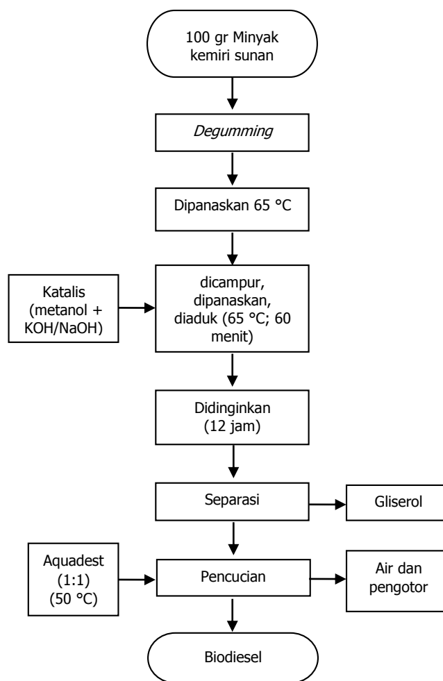
Gambar 1. Diagram proses pembuatan biodiesel dari minyak kemiri sunan
