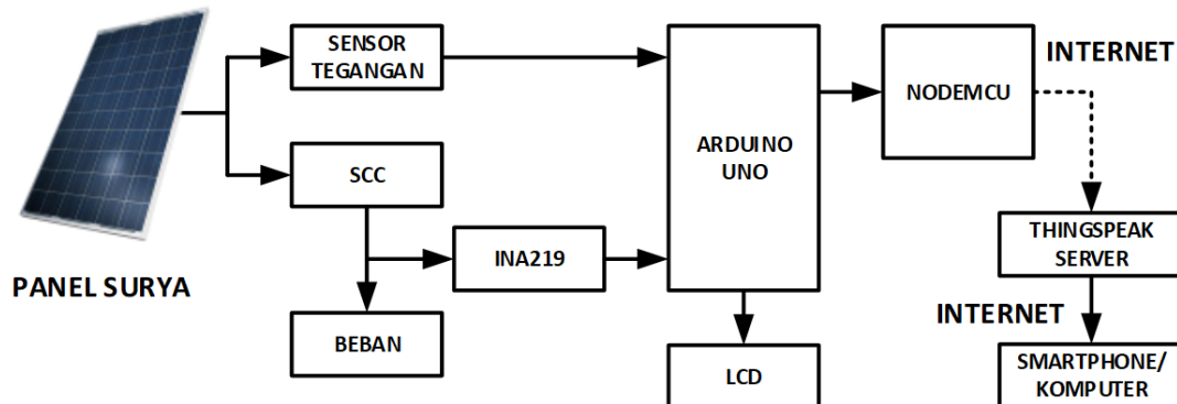
Gambar 1. Diagram blok sistem pemantauan panel surya berbasis IoT
