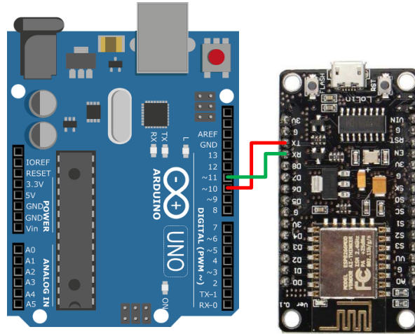
Gambar 4. Rancangan komunikasi serial dari Arduino Uno ke NodeMCU
