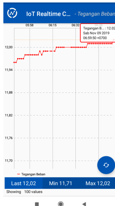
Gambar 8. Hasil tampilan pemantauan tegangan beban melalui Thingview
