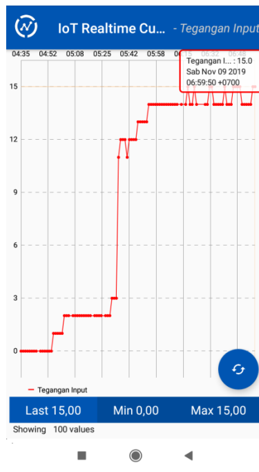
Gambar 10. Hasil tampilan pemantauan tegangan yang dihasilkan panel surya melalui Thingview
