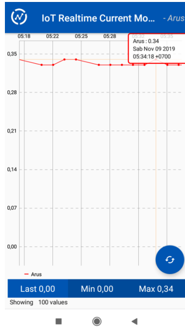
Gambar 9. Hasil tampilan pemantauan arus beban melalui Thingview
