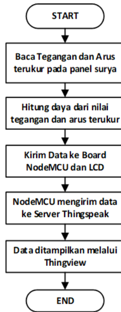
Gambar 5. Diagram alir pemantauan tegangan dan daya panel surya menggunakan IoT
