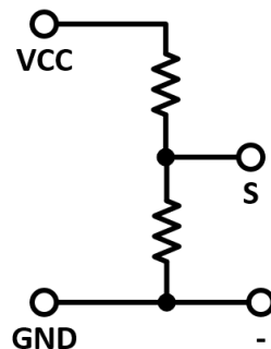
Gambar 2. Rangkaian pembagi tegangan pada modul sensor tegangan
