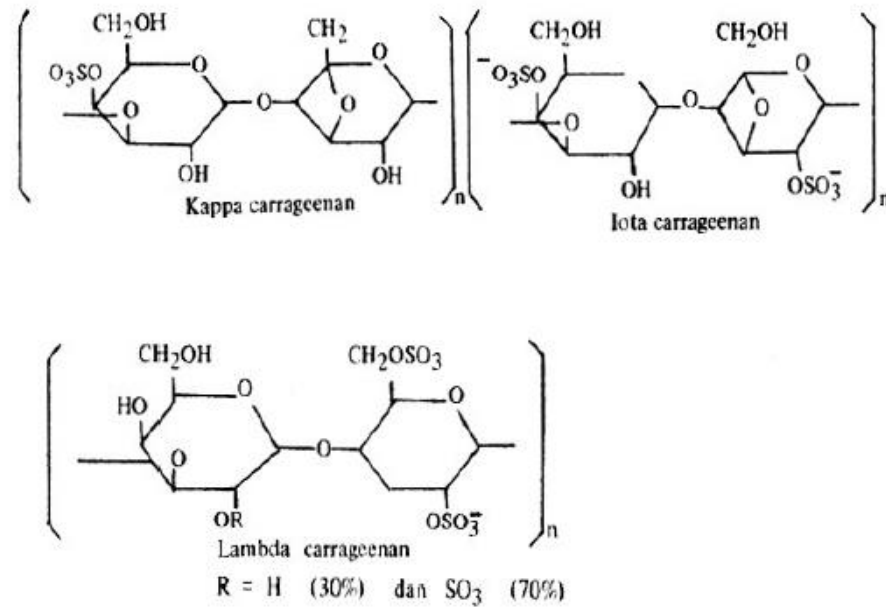
Gambar 2. Struktur Kimia Karagenan Sumber : Ulfah (2009)
