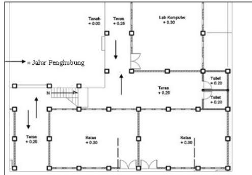
Gambar 7. Rancangan laboratorium komputer
