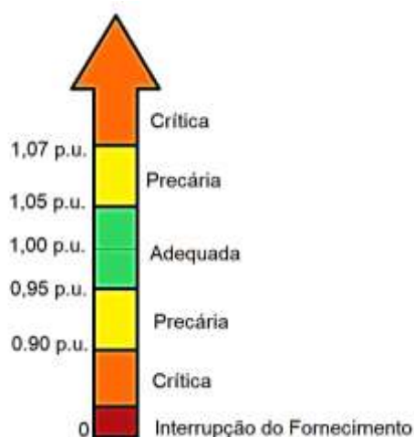
Figura 2.4 - Faixas de tensão de fornecimento entre 69 kV e 230 kV. Fonte: ANEEL (2017).
