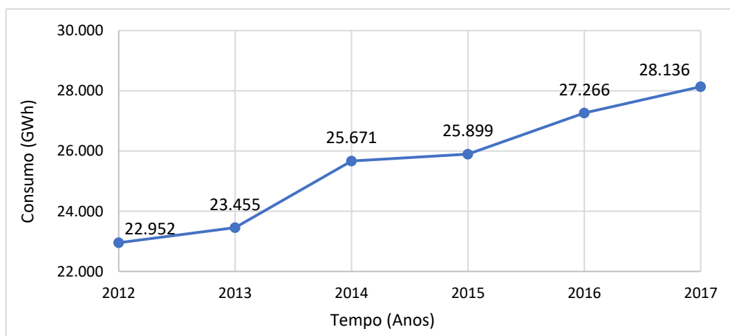
Figura 1.1 – Volume de consumo da classe rural no Brasil. Fonte: EPE (2017)
