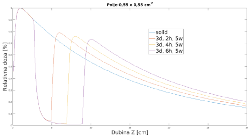
Grafik 1. PDD kriva za polje 0.55 x 0.55 cm 2 , i vazdušnu šupljinu pozicioniranu na 3 cm, površine 5 cm 2 , i variranih visina od 2 cm, 4 cm, 6 cm.
