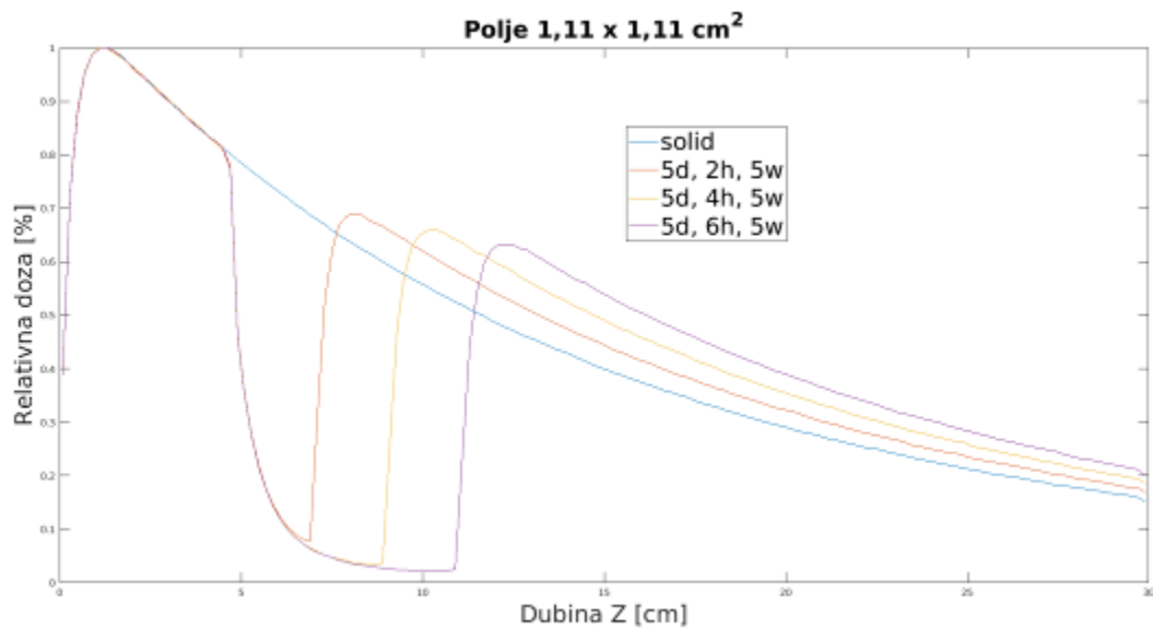
Grafik 2. PDD kriva za polje 1.11 x 1.11 cm 2 , i vazdušnu šupljinu pozicioniranu na 5 cm, površine 5 cm 2 , i variranih visina od 2 cm, 4 cm, 6 cm.
