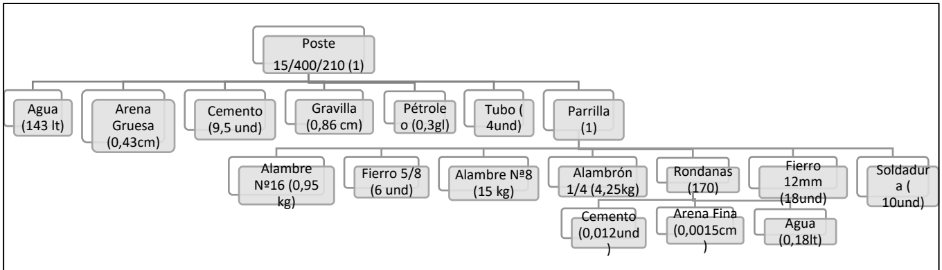
ANEXO 45: Ilustración 10 Lista estructurada de materiales: Poste de 15/400/2/210/435
