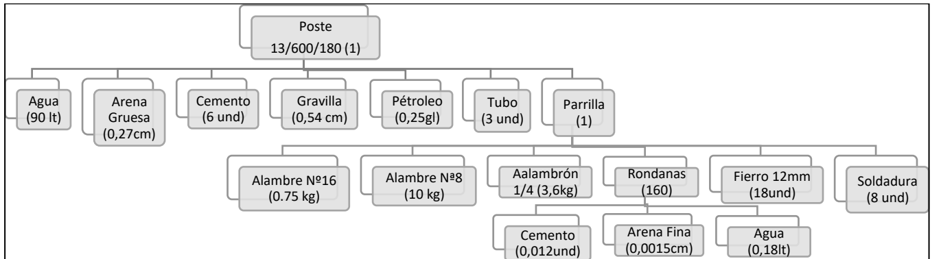
ANEXO 41: Ilustración 6 Lista estructurada de materiales: Poste de 13/600/2/180/375
