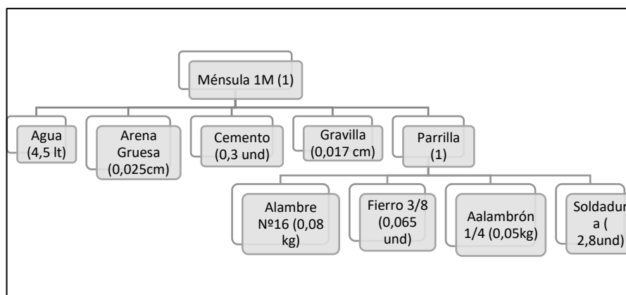
Ilustración 15: Lista estructurada de materiales: Ménsula de 1M
