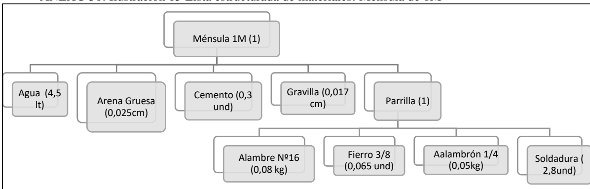
ANEXO 50: Ilustración 15 Lista estructurada de materiales: Ménsula de 1M
