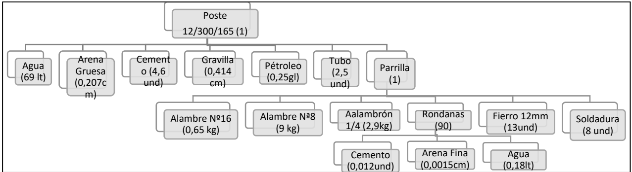
ANEXO 51: Ilustración 16 Lista estructurada de materiales: Poste de 12/300/2/165/345
