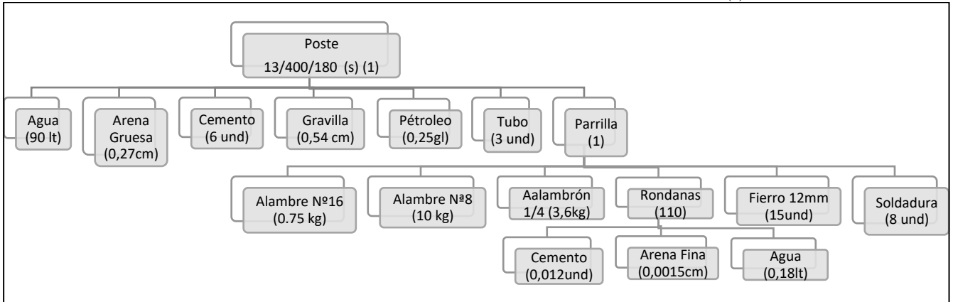
ANEXO 52: Ilustración 17 Lista estructurada de materiales: Poste de 13/400/2/180/375 (s)
