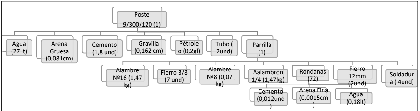
ANEXO 37: Ilustración 2 Lista estructurada de materiales: Poste de 9/300/2/120/255
