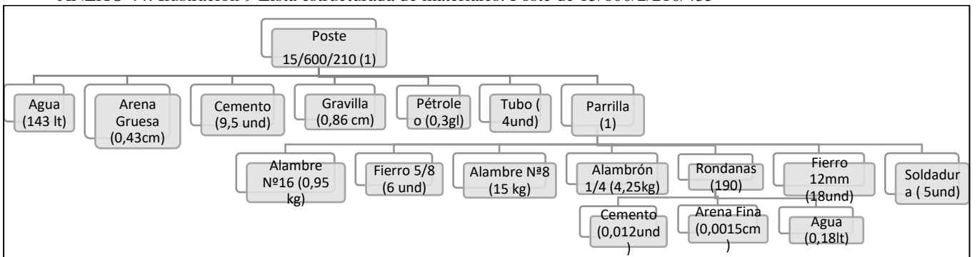
ANEXO 44: Ilustración 9 Lista estructurada de materiales: Poste de 15/600/2/210/435
