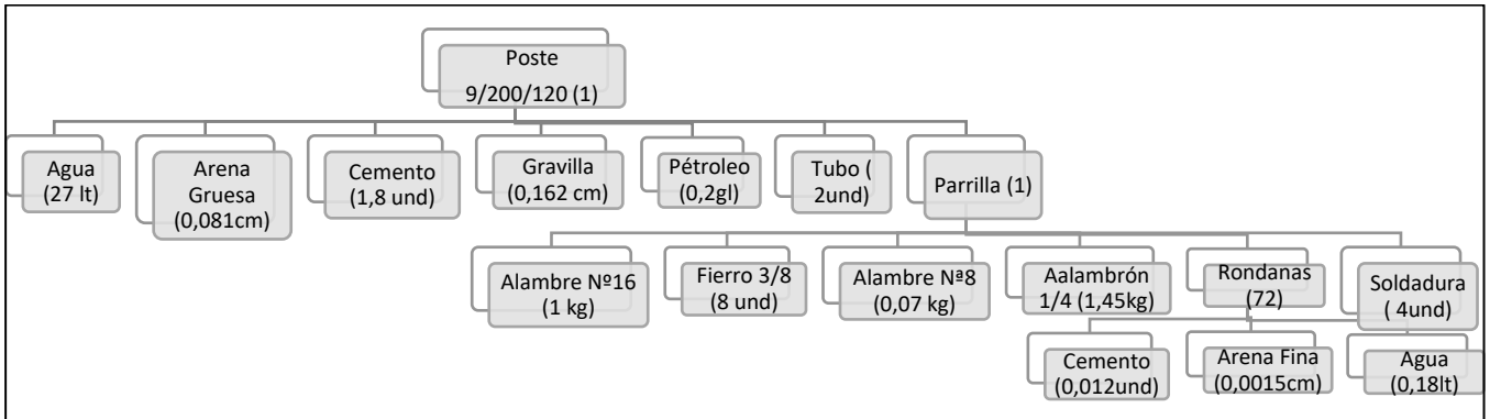
ANEXO 38: Ilustración 3 Lista estructurada de materiales: Poste de 9/200/2/120/255
