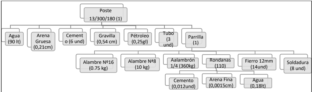
ANEXO 36: Ilustración 1 Lista estructurada de materiales: Poste de 13/300/2/180/375
