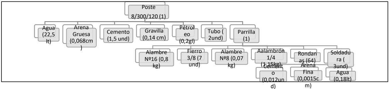
ANEXO 49: Ilustración 14 Lista estructurada de materiales: Poste de 08/300/2/120/240
