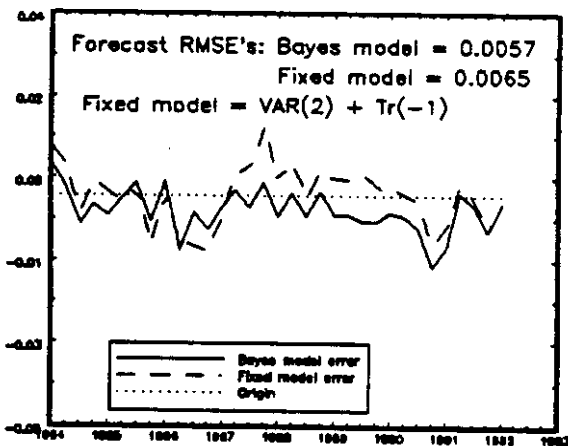
Figure 15: GDP: 1959:1–1992:1
