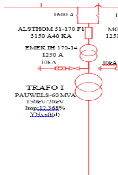
Gambar 3. Single line diagram arrester dengan trafo 1
