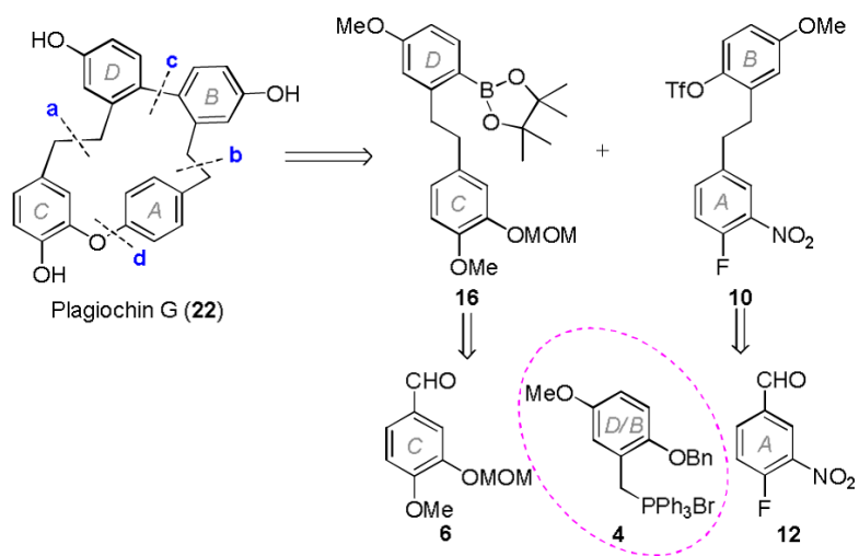
Scheme 1. Retrosynthetic analysis of plagiochin G.
