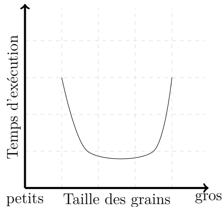
Figure 2.7 Courbe illustrant l'effet général de la taille des grains (des tâches) sur le temps d'exécution. Inspiré de Tremblay [47].
