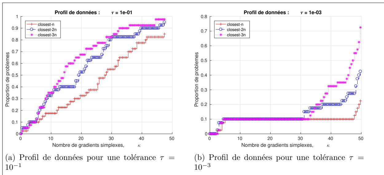
Figure 5.7 Comparaison des performances de PCA-MADS avec différents nombres des plus proches points sélectionnés pour l'analyse de sensibilité (stratégie closest - n ), sur une partie de la suite de fonctions bbob-largescale de COCO
