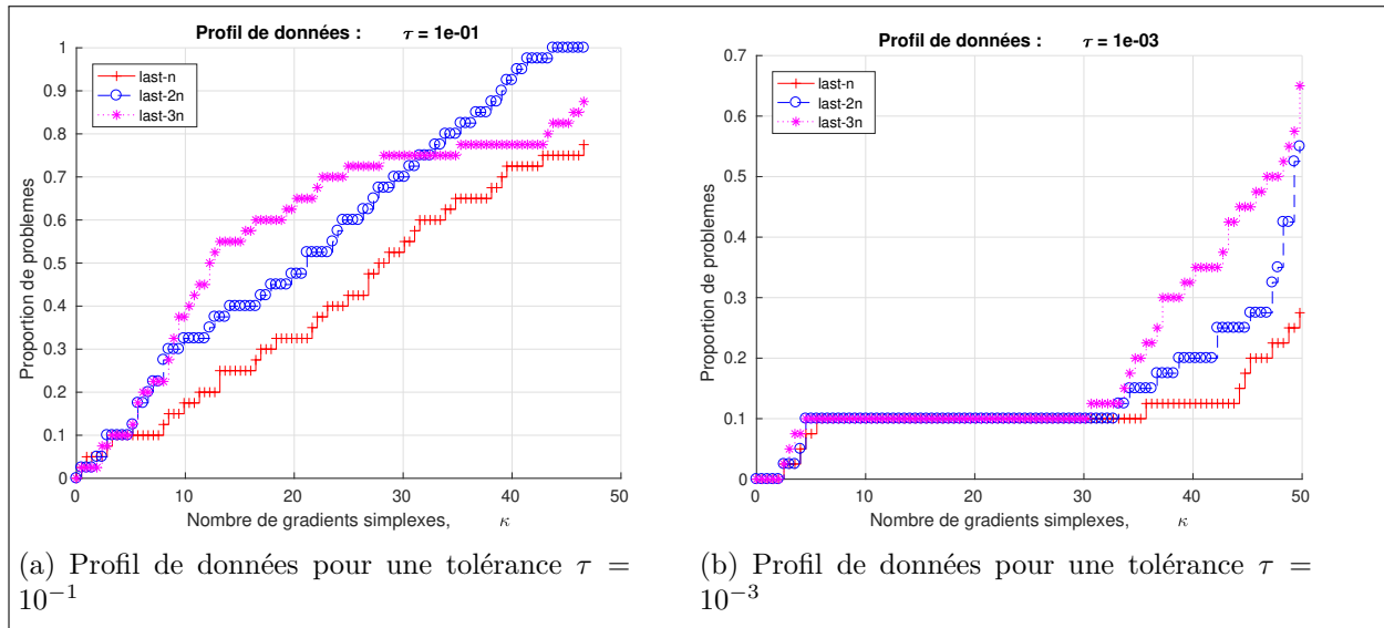
Figure 5.6 Comparaison des performances de PCA-MADS avec différents nombres des derniers points sélectionnés pour l'analyse de sensibilité (stratégies last - n ), sur une partie de la suite de fonctions bbob-largescale de COCO
