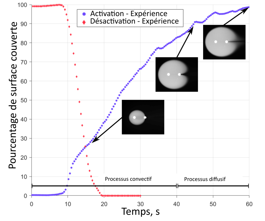
Figure 5.15 Cinétiques expérimentales de l'établissement et de l'interruption du confinement. Pour l'activation, l'axe des ordonnées correspond à la part de la surface "finale" (camouflage stationnaire à t = +\infty ) couverte par le camouflage en cours d'établissement. Pour la désactivation, l'axe des ordonnées correspond à la part de la surface "initiale" (camouflage stationnaire à t < 0s ) couverte par le camouflage en cours d'interruption.
