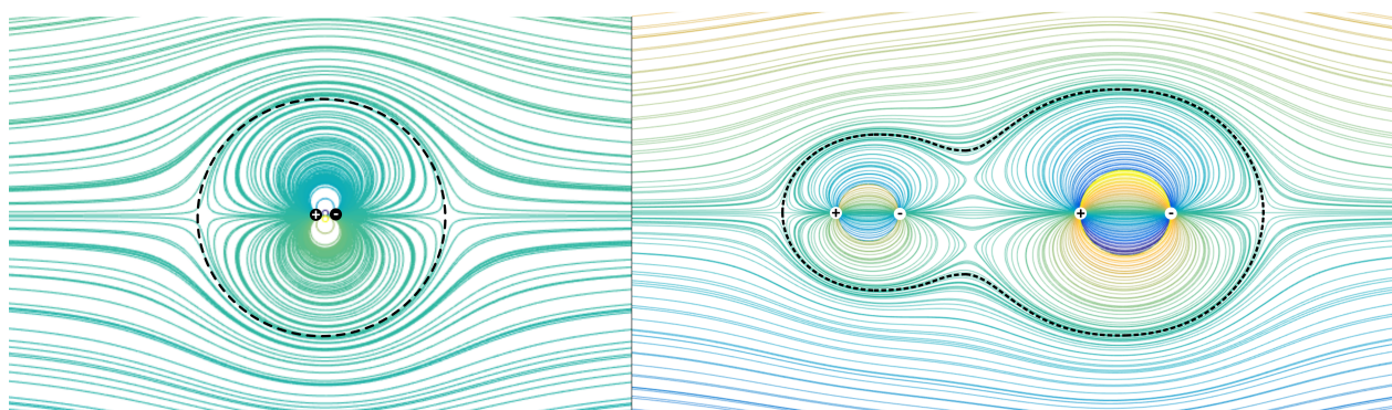
Figure 2.3 Exemples de corps de Rankine, tracés sur matlab par Oscar Boyadjian. Les lignes pleines correspondent aux lignes de courant de l'écoulement, les lignes pointillées au contour du corps de Rankine. Les signes + et - désignent respectivement une injection et une aspiration. À gauche, le corps de Rankine le plus célèbre : le cercle, formé avec deux ouvertures infiniment proches. À droite, exemple d'un corps de Rankine plus complexe réalisé avec 4 ouvertures.
