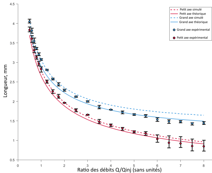
Figure 5.6 Petits et grands axes du camouflé en fonction de \frac{Q}{Q_{inj}} . Les barres d'erreur désignent les valeurs minimales et maximales mesurées.
