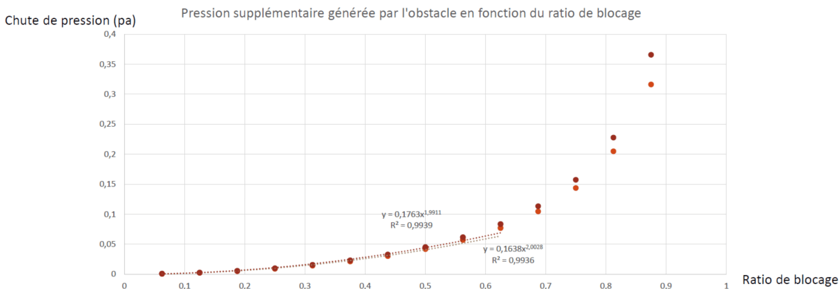
Figure 3.3 Chutes de pression supplémentaires générées par un obstacle en fonction du ratio de blocage. En rouge sombre, le cas où l'obstacle adhère et en orange le cas où il glisse (dans les deux cas, les murs latéraux adhèrent).
