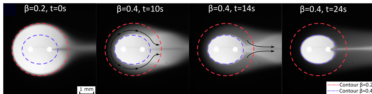
Figure 5.16 Réponse expérimentale du camoufflage lorsque Q/Q_{inj} est brutalement augmenté de 1 à 2.
