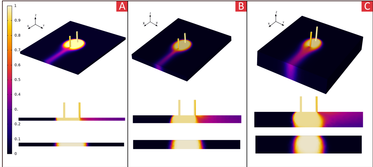
Figure 4.1 Visualisation de l'influence de G par cartes de concentration simulées. (A) Cas où G = 200\mu m . De haut en bas : vue en perspective de la simulation 3D, coupe du confinement en son centre selon l'axe x , coupe du confinement en son centre selon l'axe y . La barre à gauche est la légende de couleur pour les cadrans A, B et C. (B) Cas G = 500\mu m . (C) Cas G = 1mm .
