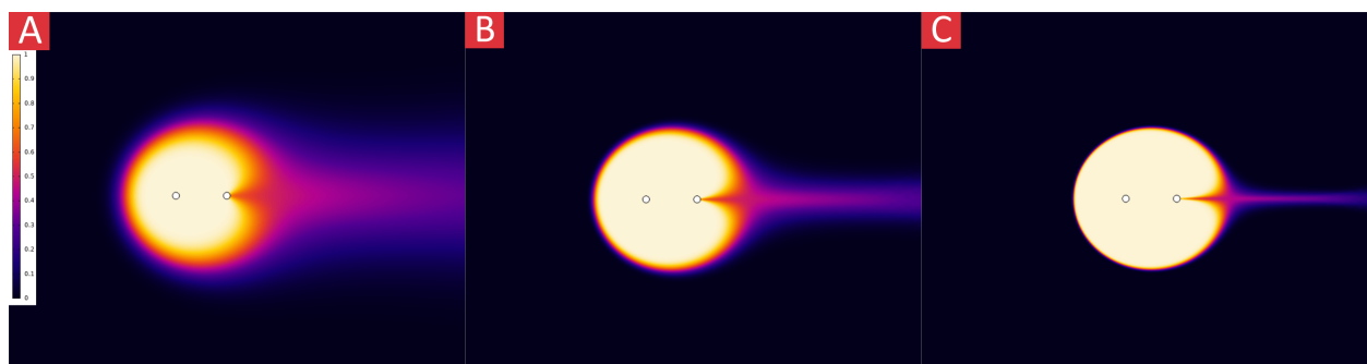
Figure 4.5 Visualisation de l'influence du nombre de Péclet par cartes de concentration simulées en 2D. (A) Cas où Pe = 65 . Les disques blancs correspondent aux ouvertures. La barre à gauche est la légende de couleur pour les cadrans A, B et C. (B) Cas Pe = 655 . (C) Cas Pe = 6556 .
