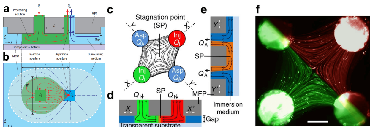
Figure 2.2 Exemples de dispositifs microfluidiques ouverts. (a) et (b) Schémas selon plusieurs vues d'une MFP, reproduits de [11] avec la permission de Springer Nature. (c), (d) et (e) Schémas selon plusieurs vues d'un quadrupôle microfluidique, et (f) une réalisation expérimentale de celui-ci. Reproductions de [53] avec la permission de Springer Nature.
