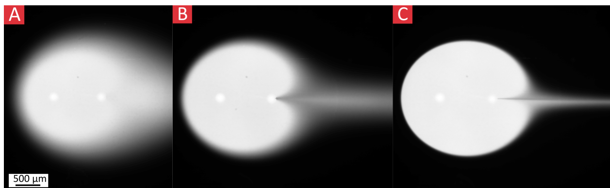
Figure 5.8 Exemples du même dispositif à différents nombres de Péclet global. Pe_A = 26 , Pe_B = 260 , Pe_C = 2600 . La barre d'échelle est commune à tous les panneaux.
