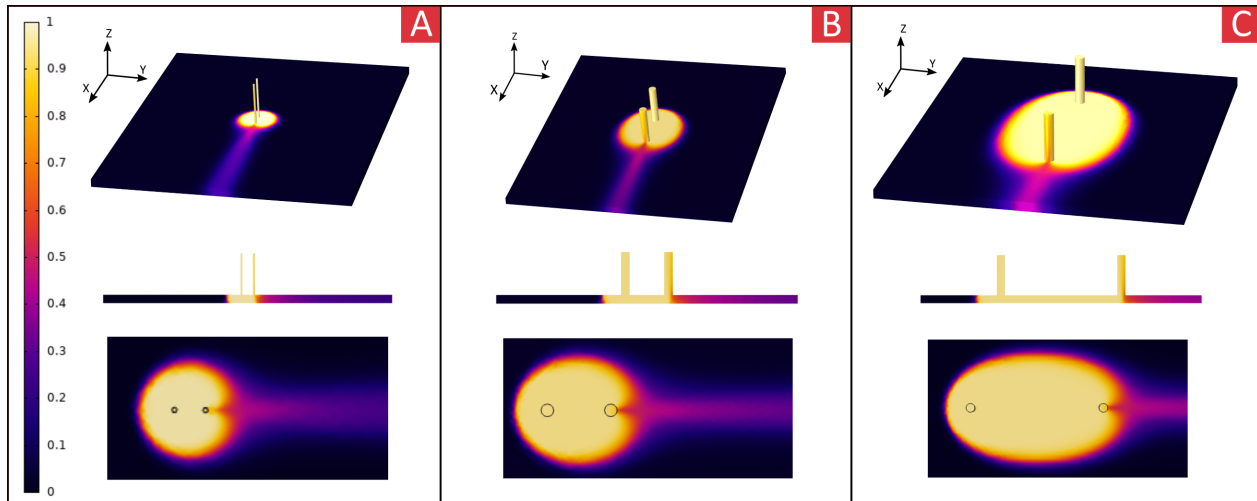
Figure 4.3 Visualisation de l'influence du ratio \frac{d}{W} par cartes de concentration simulées. (A) Cas où \frac{d}{W} = 0.05 . De haut en bas : vue en perspective de la simulation 3D, coupe du confinement en son centre selon l'axe x , vue du dessus du confinement. Les cercles noirs correspondent aux ouvertures. La barre à gauche est la légende de couleur pour les cadrans A, B et C. (B) Cas \frac{d}{W} = 0.16 . (C) Cas \frac{d}{W} = 0.5 .
