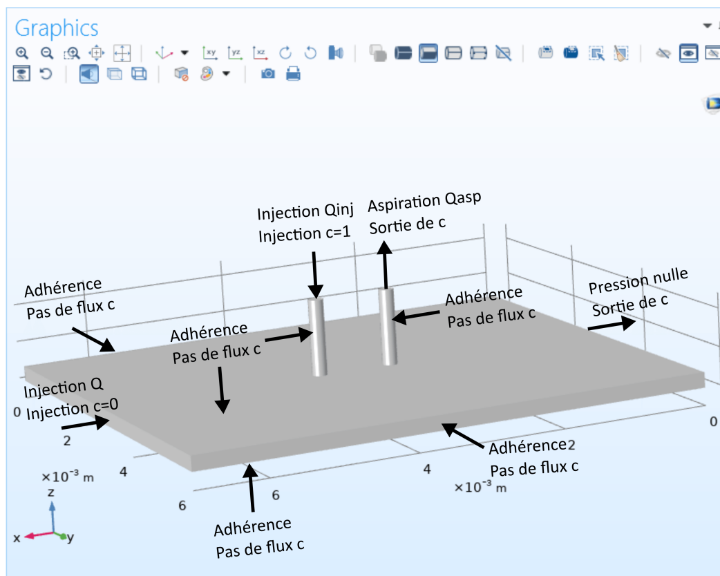
Figure B.1 Conditions aux limites imposées sur le modèle COMSOL. La première ligne fait référence à l'écoulement, la deuxième ligne au transport d'espèces, c désignant la concentration.
