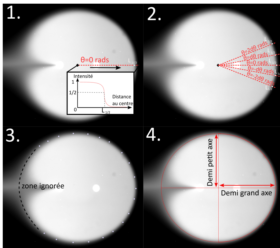
Figure D.1 Schéma de fonctionnement du code permettant l'obtention de la forme du corps de Rankine à partir de la carte de concentration expérimentales.
