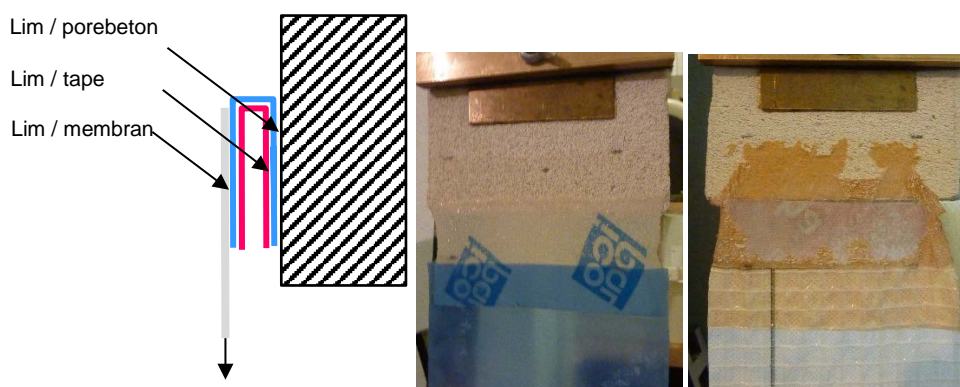
FIGUR 10. Forskellige steder klæbningen kunne svigte, når membran blev trukket af porebeton. Tv. Her er tapen fremstillet som to lag, dels selve limen, der er vist med blå, dels bærelaget, der er vist med rødt. Th. To fotos der viser forskellige steder klæbningen kan bryde, dels et hvor porebetonen næsten er ren, derfor er bruddet sket mellem lim og porebeton, dels en hvor tapens bærelag er næsten rent, derfor er bruddet sket mellem lim og tape.
