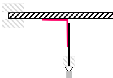
FIGUR 18. Skematisk fremstilling af afprøvning af aftrækningsstyrke ved 90°, hvor membran er klæbet på bøgetræ. Metoden er ikke benyttet i dette projekt, men beskrives i udkast til DIN 4108-11 (2016). Opstillingen placeres i varmeskab ved 40 °C i 24 timer med et lod for enden af membranen.
