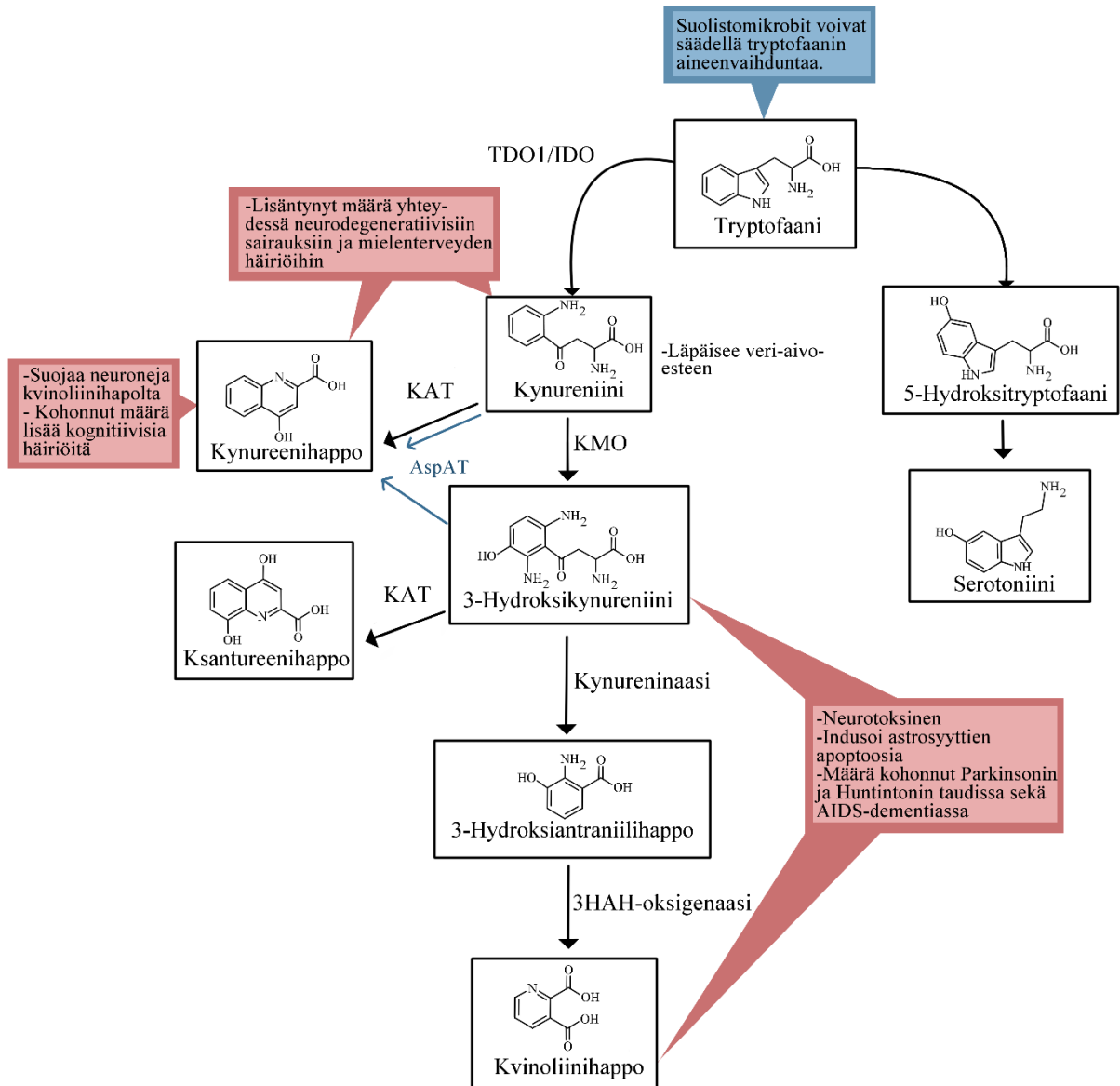
Kuva 7. Kynureeniinireitti. Tryptofaania voidaan muuntaa mm. kynureeniinireitin aineenvaihduntatuotteiksi sekä serotoniiniksi (Kennedy et al., 2017). TDO: tryptofaani-2,3-dioksigenaasi, IDO1: indoliamiini-2,3-dioksigenaasi, KAT: kynureeniiniaminotransferaasi, KMO: kynureeniini-3-mono-oksigenaasi, 3HAH: 3-hydroksiantraniilihappo, AspAT: aspartaattiaminotransferaasi. AspAT-entsyymiä esiintyy mm. kolibakteereissa.
