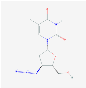
Kuva 3. AZT:n rakennekaava (Kim S et al. 2018. Pubchem)
