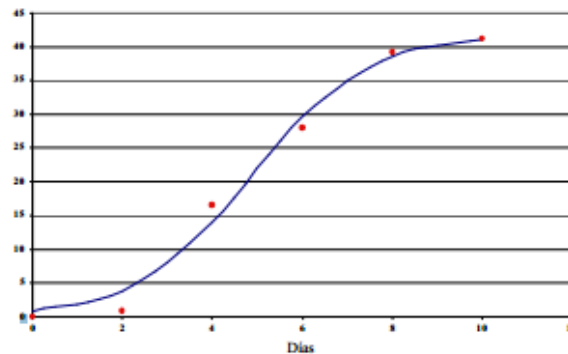
Figura 2. Tiempo de maduración típica de biofiltros en base a las concentraciones de N-NO 3 (Sonnenholzner, 2004)
