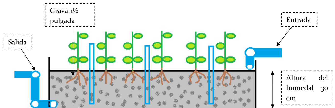
Figura 4. Diseño de los humedales a evaluarse.
