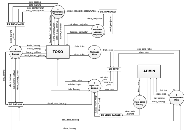
Gambar 2 Rancangan DFD
