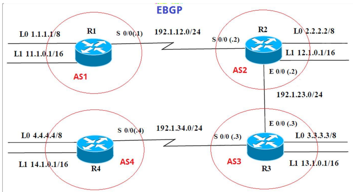
Figura 17. Topología Escenario 2
