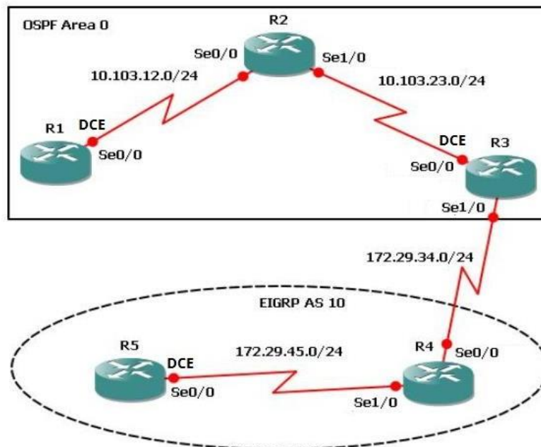
Figura 1. Topología Escenario 1
