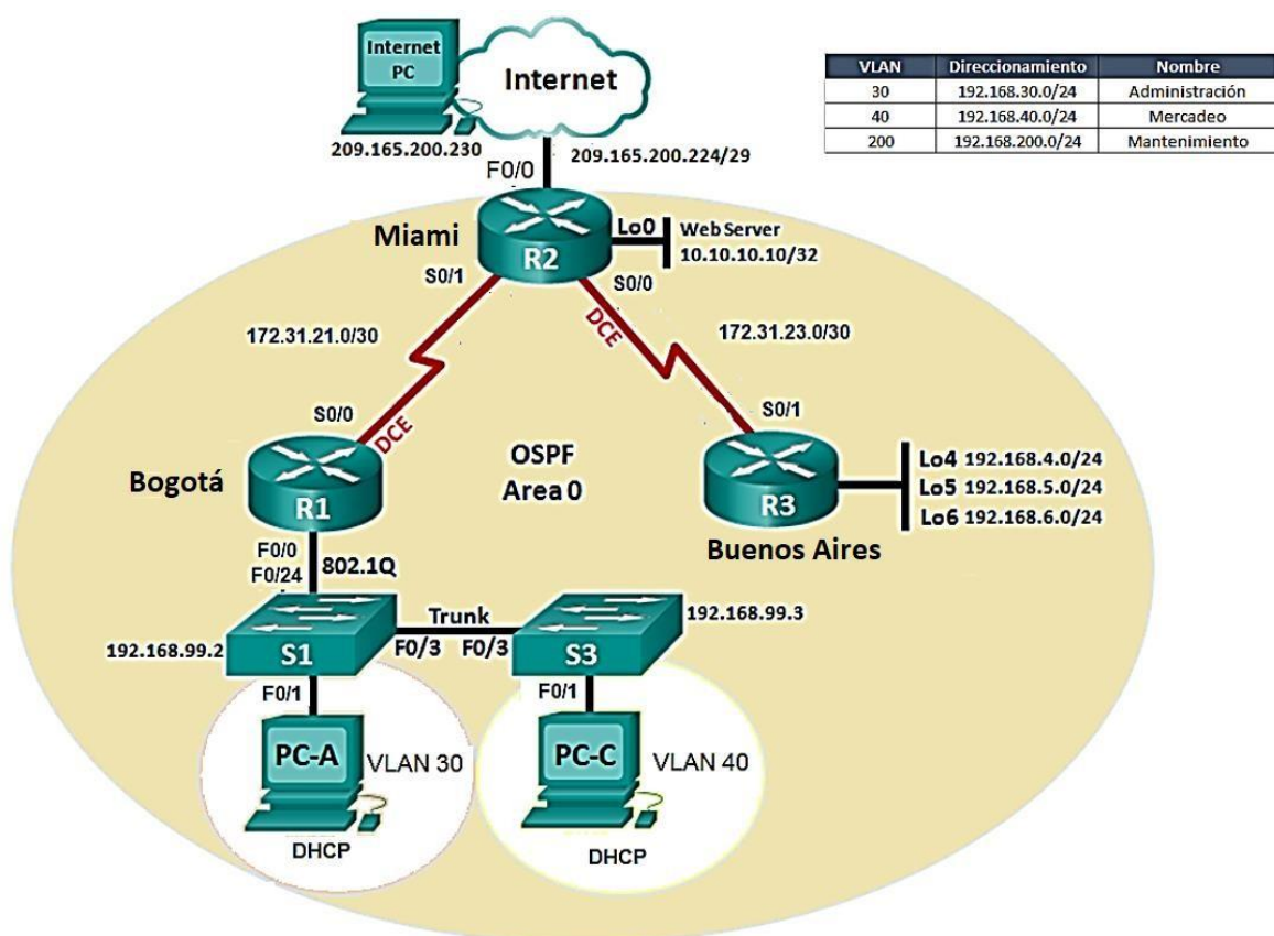
Imagen 24 Escenario 2
