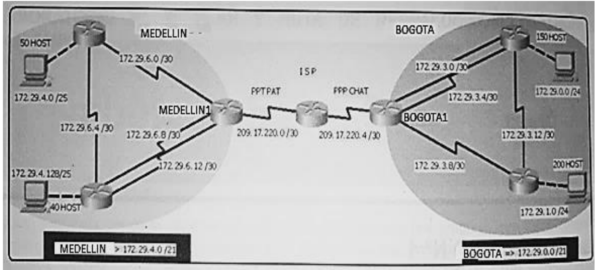
Imagen 1 Topología Escenario 1
