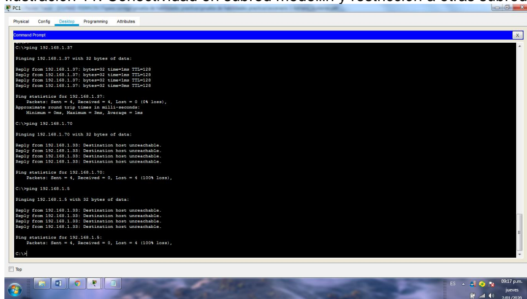
Ilustración 11: Conectividad en subred medellin y restricción a otras subredes
