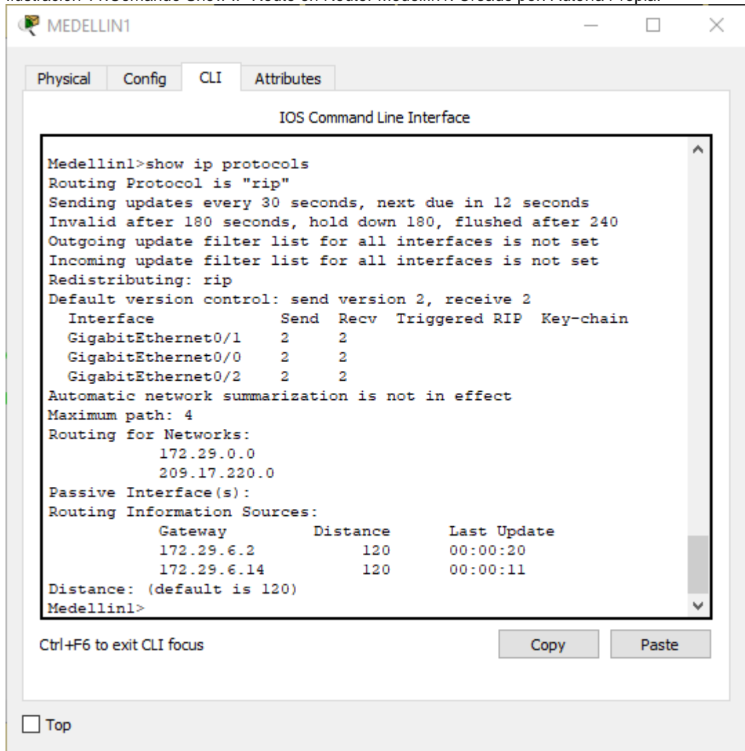
Ilustración 11. Comando Show IP Route en Router Medellín1. Creado por: Autoría Propia.
