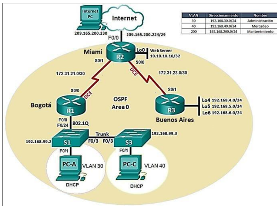
Ilustración 14 Administración de red escenario 2-A
