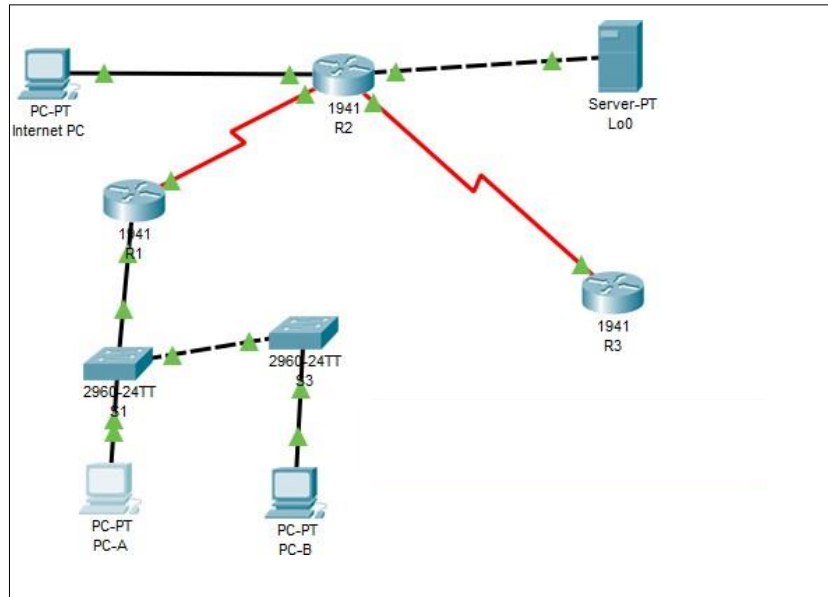
Ilustración 15 Administración de red escenario 2-B
