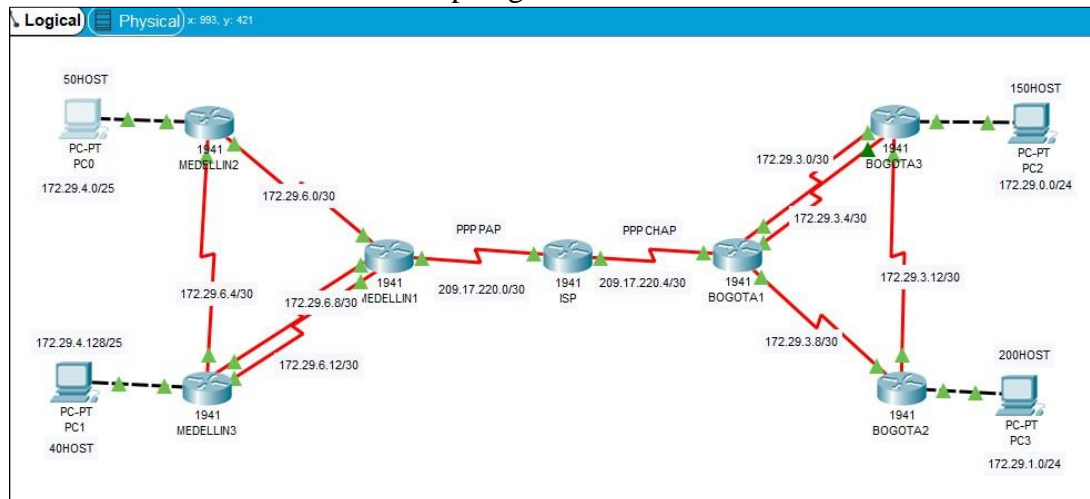
Ilustración 2 Tipología de Red II
