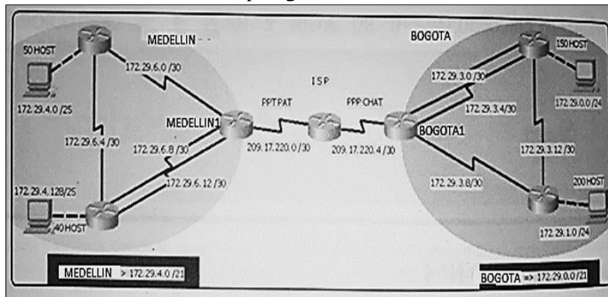
Ilustración 1 Tipología de Red I
