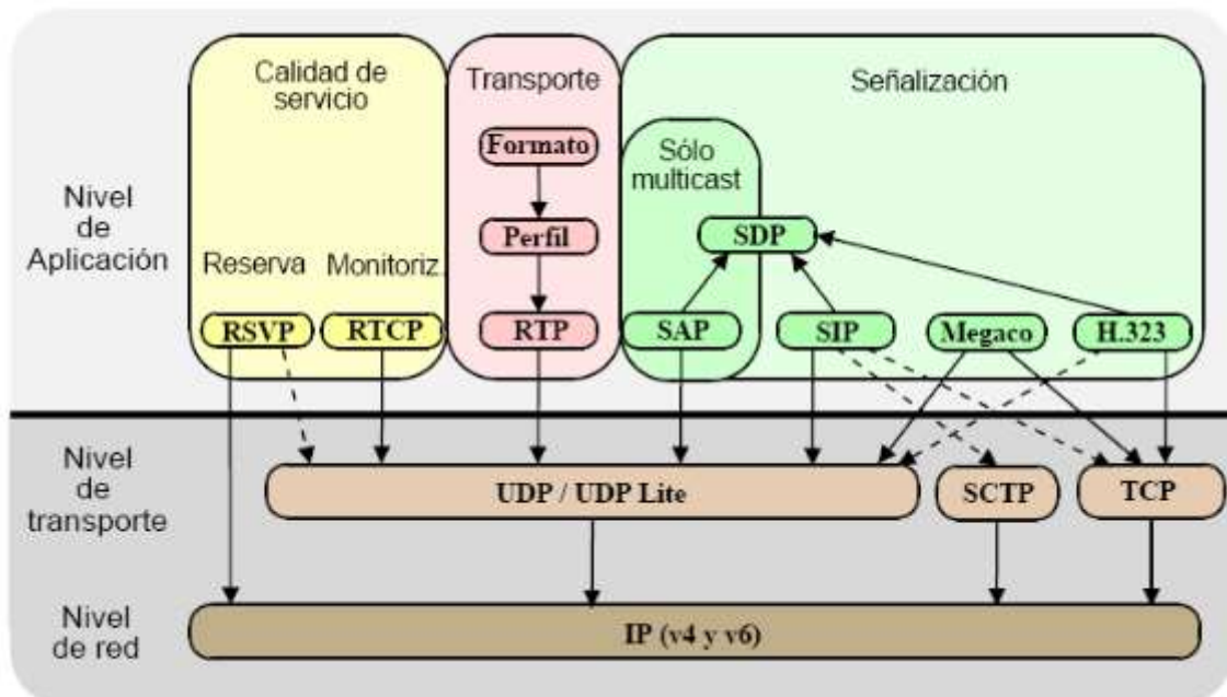
Figura 2. Funcionamiento de un servidor VoIP. (prosciencas, 2019)
