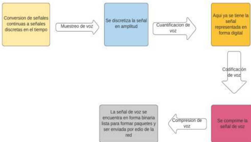
Figura 1. Funcionamiento de un servidor VoIP. (Carrillo, 2019)
