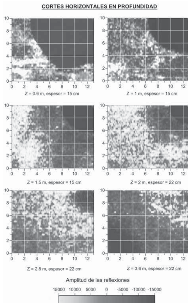
Figura 17. Cortes horizontales obtenidos a partir de la exploración con georradar del sector RADAR-2.
