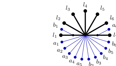
(d) After adding \pi_8 = [12346|57]
