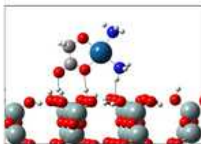
G2 \Delta E = -3.30 eV
