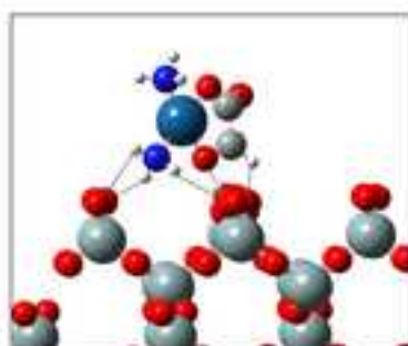
G5 \Delta E = -8.99 eV
