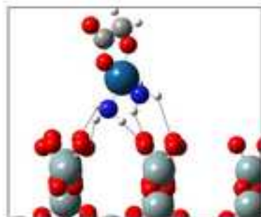
G3 \Delta E = -7.03 eV
