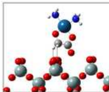
G4 \Delta E = -5.97 eV
