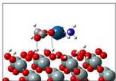
G1 \Delta E = -2.62 eV
