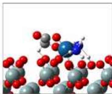
G1 \Delta E = -9.07 eV
