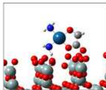
G2 \Delta E = -7.09 eV
