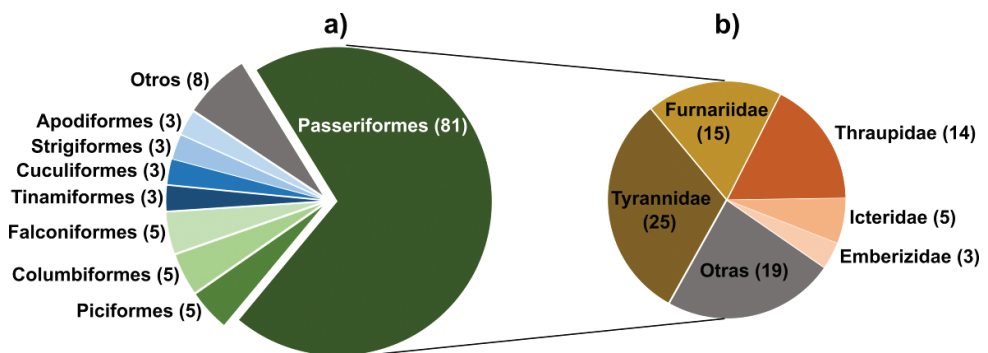
Figura 3. Órdenes y familias de aves muestreadas en el área de estudio, en la provincia fitogeográfica del Espinal, Argentina: a) proporciones en las que se encuentran representados los órdenes en función al número de especies incluidas en cada uno de ellos; b) proporciones en las que se encuentra representada cada una de las familias del orden Passeriformes en función al número de especies. Los números entre paréntesis indican el número de especies incluidas en cada orden (a) y en cada familia (b).
