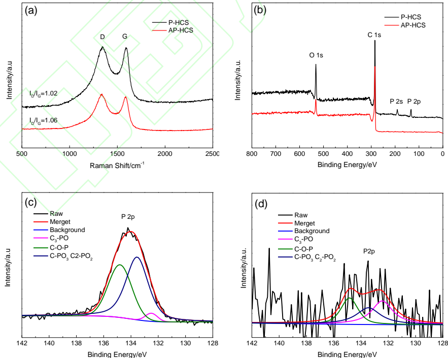
图4 P-HCS 和 AP-HCS 的 Raman 光谱图 (a)、XPS 全谱 (b); P-HCS 和 AP-HCS 的 P2p 高分辨谱 (c) (d) Fig.4 Raman spectra (a) and XPS survey spectra (b) of P-HCS and AP-HCS; P2p XPS spectra of P-HCS and AP-HCS (c) (d)
