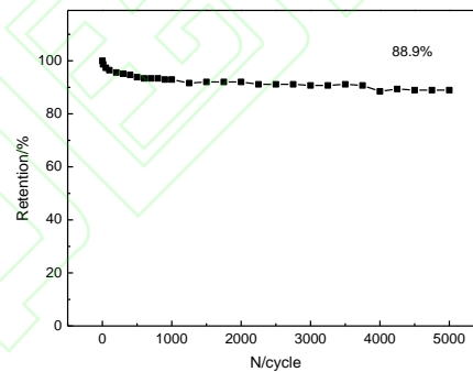
图 7 AP-HCS 在电流密度为 5A/g 下的循环性能
