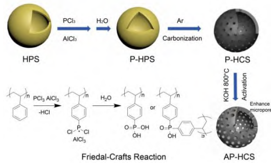
图 1 中空碳球 AP-HCS 的制备过程
