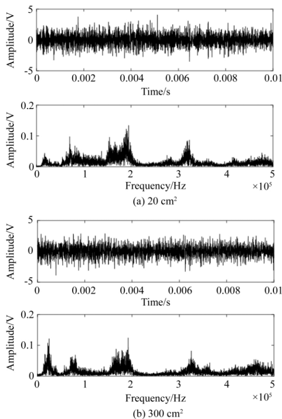
图 2 声发射信号的时域波形与频谱
