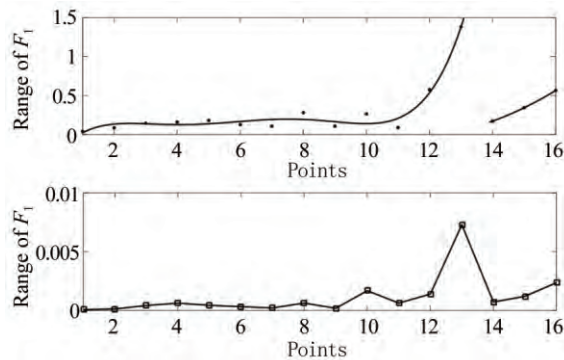
图 5 砂轮磨损曲线
