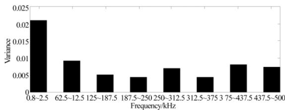
图 3 小波包能量谱系数方差
