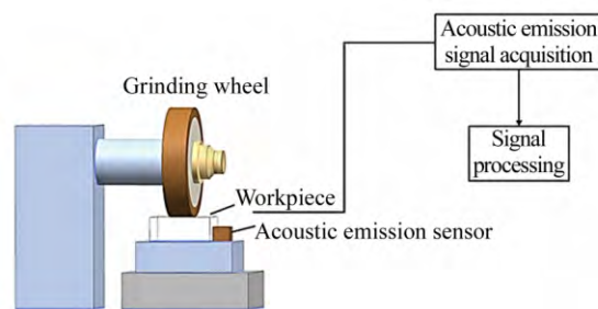
图 1 砂轮磨损监测实验装置
