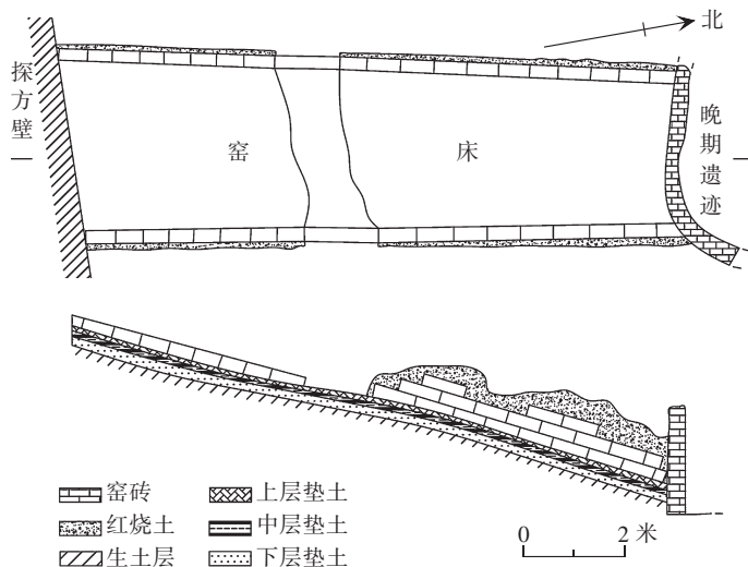
图五 2017YPSY1 平、剖面图
