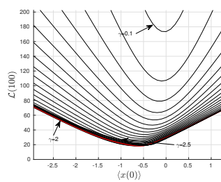
(d) Zoom-in of panel (c).
