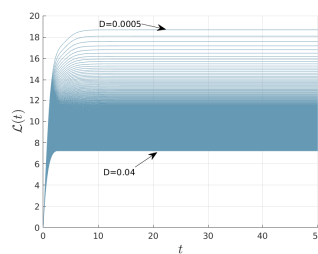
(d) Time-evolution of \mathcal{L}(t) .
