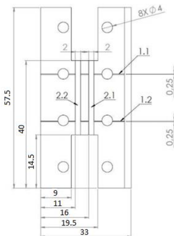
Slika 17. Ispitni uzorak 1. [14]
